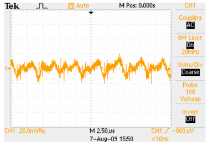
Noise V_{IN}=12V , I_O=16A , 5~20MHz Bandwidth
