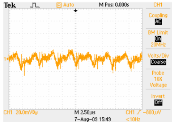
Noise V_{IN}=12V , I_O=16A , 5~20MHz Bandwidth
