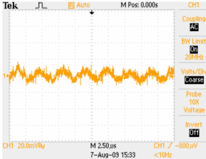
Noise V_{IN}=5V , I_O=16A , 5~20MHz Bandwidth
