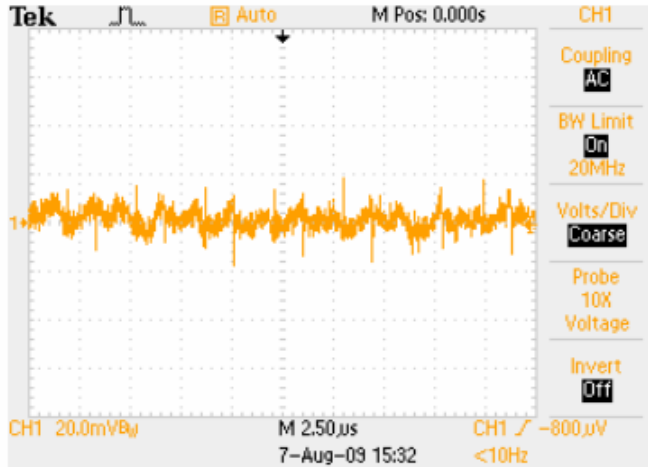
Noise V_{IN}=5V , I_O=16A , 5~20MHz Bandwidth
