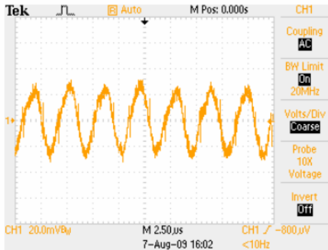
Noise V_{IN}=12V , I_O=16A , 5~20MHz Bandwidth
