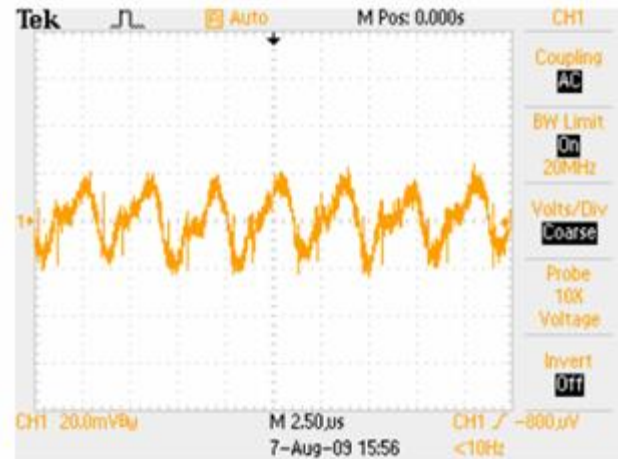
Noise V_{IN}=12V , I_O=16A , 5~20MHz Bandwidth
