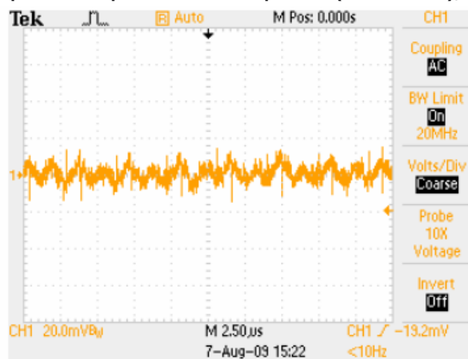
Noise V_{IN}=5V , I_O=16A , 5~20MHz Bandwidth
