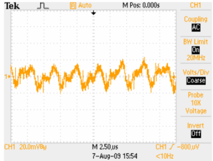
Noise V_{IN}=12V , I_O=16A , 5~20MHz Bandwidth
