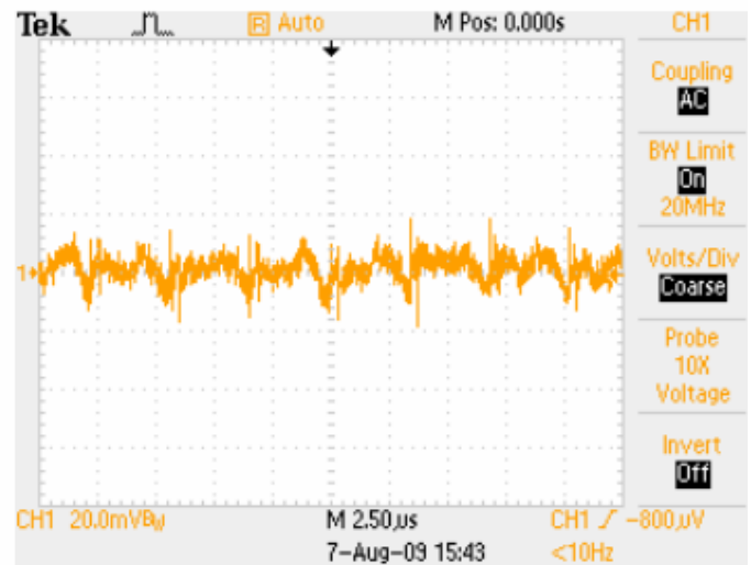
Noise V_{IN}=11V , I_O=16A , 5~20MHz Bandwidth
