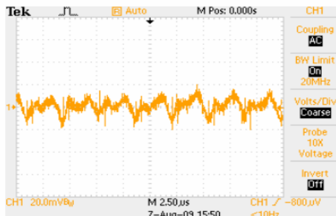
纹波与噪声: 输入 12V, 16A 负载, 5~20MHz 带宽
