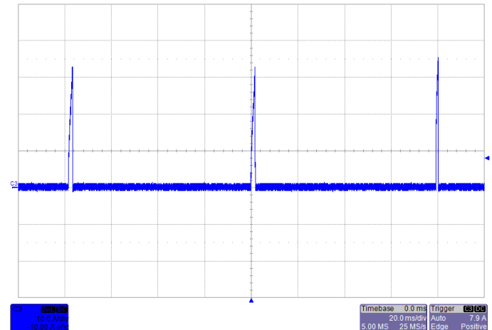
输出短路电流波形，输入电压 12V
