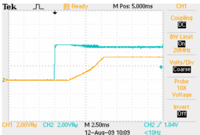
启动波形: 输入 5V, 负载 16A 黄色: 输出电压; 蓝色: 输入电压
