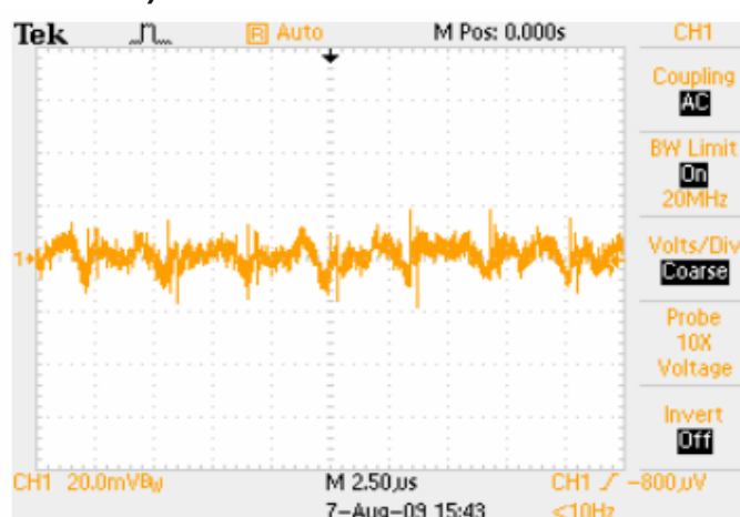
纹波与噪声: 输入 11V, 16A 负载, 5~20MHz 带宽
