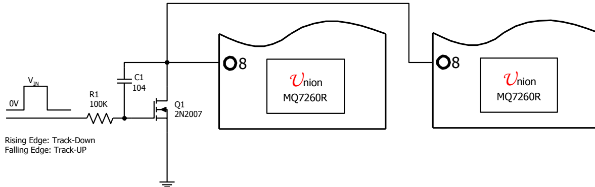
图三，使用EasyTrack™同时上电和下电电路
