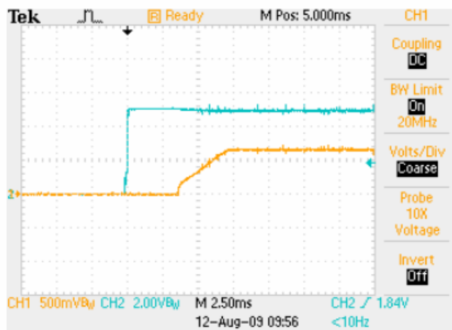
启动波形: 输入 5V, 负载 16A 黄色: 输出电压; 蓝色: 输入电压
