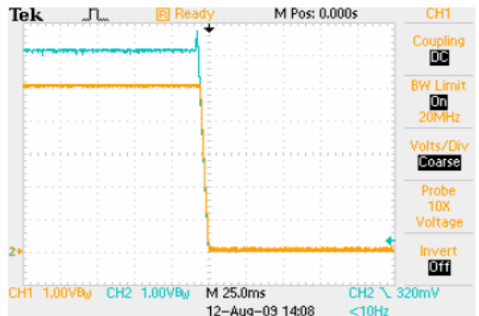
用 EasyTrack™ 控制下电过程, 控制压 12V, 负载 16A 蓝色: EasyTrack™ 控制电压 黄色: 输出电压
