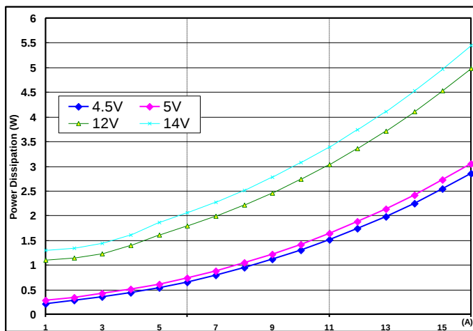
功率损耗 vs. 负载电流
