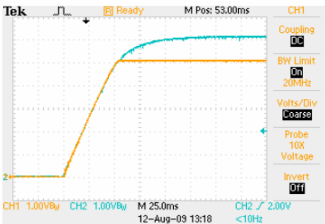
用 EasyTrack™ 控制上电过程, 控制压 12V, 负载 16A 蓝色: EasyTrack™ 控制电压 黄色: 输出电压
