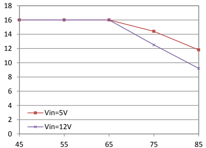
输出电流降额 (自然冷却)
