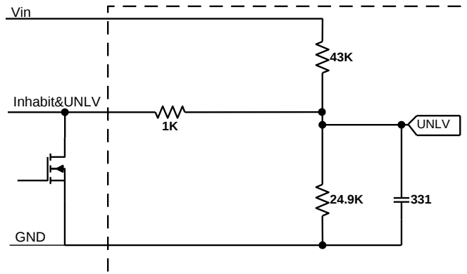
图 5, 用集电极和漏极开路晶体管实现输出的开或关
