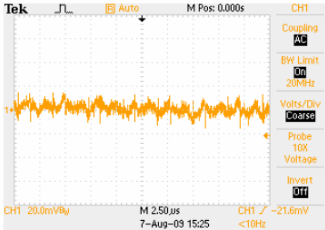
纹波与噪声: 输入 5V, 16A 负载, 5~20MHz 带宽
