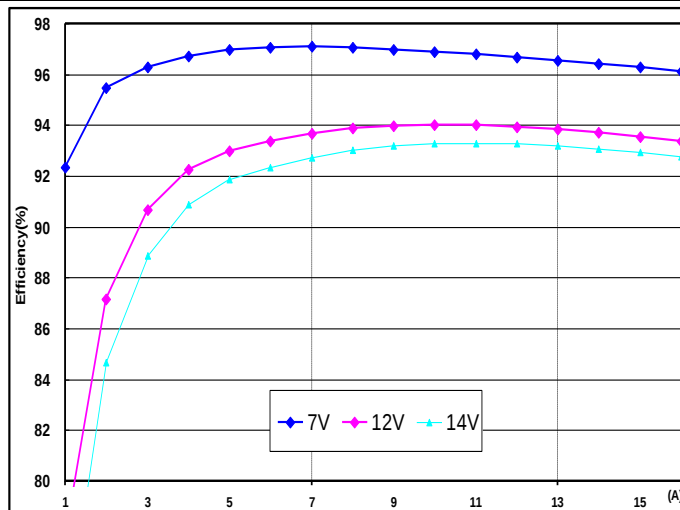
转换效率 vs. 负载电流
