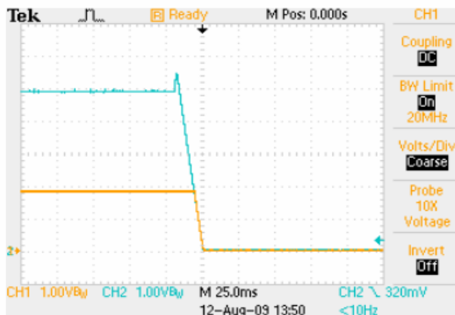
用 EasyTrack™ 控制下电过程, 控制压 5V, 负载 16A 蓝色: EasyTrack™ 控制电压 黄色: 输出电压
