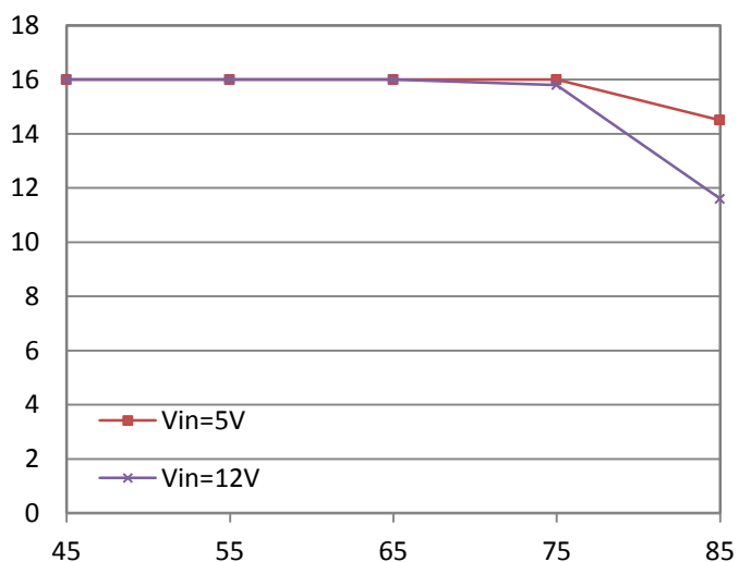
输出电流降额 (自然冷却)
