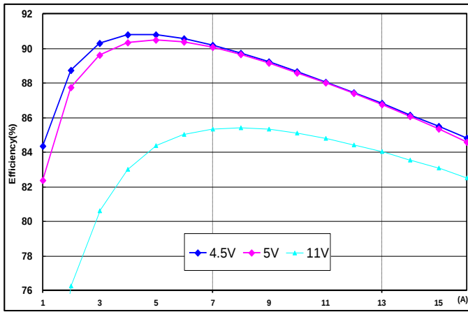
转换效率 vs.负载电流
