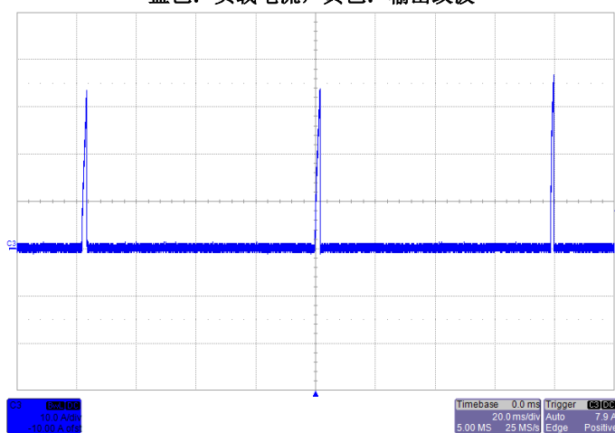
输出短路电流波形，输入电压 12V
