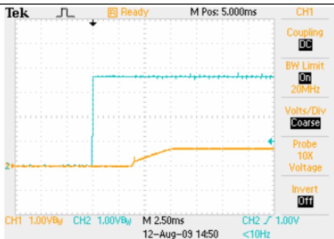
用 ON/OFF 控制上电过程, 控制压 5V, 负载 16A 蓝色: ON/OFF 控制电压 黄色: 输出电压
