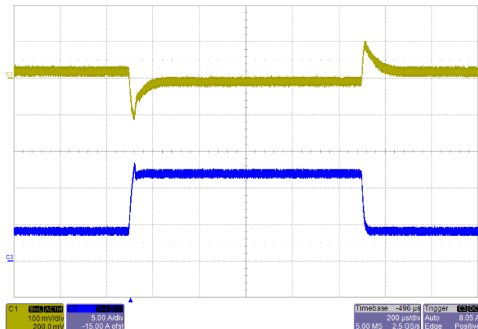
瞬态响应, 输入 5V, 阶跃 4A~12A~4A, 输出电容 220 \mu F 蓝色: 负载电流, 黄色: 输出纹波
