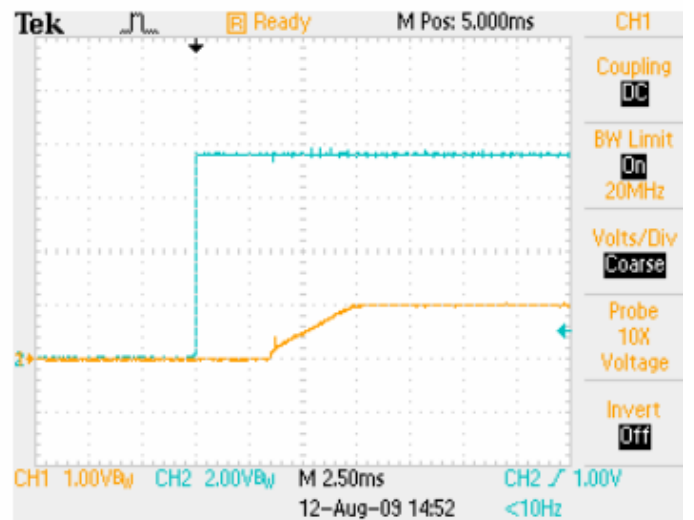
用 ON/OFF 控制上电过程，控制压 11V，负载 16A 蓝色：ON/OFF 控制电压 黄色：输出电压
