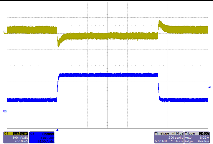
瞬态响应，输入 12V，阶跃 4A~12A~4A，输出电容 220 \mu F 蓝色：负载电流，黄色：输出纹波
