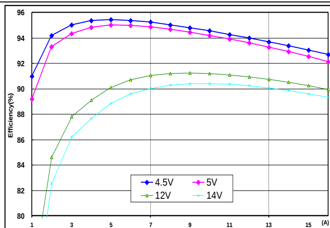
转换效率 vs. 负载电流
