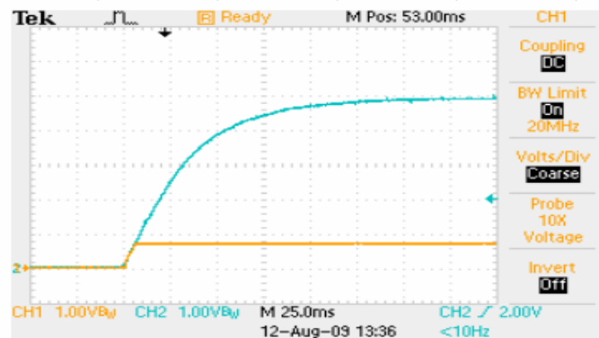
用 EasyTrack™ 控制上电过程, 控制压 5V, 负载 16A 蓝色: EasyTrack™ 控制电压 黄色: 输出电压
