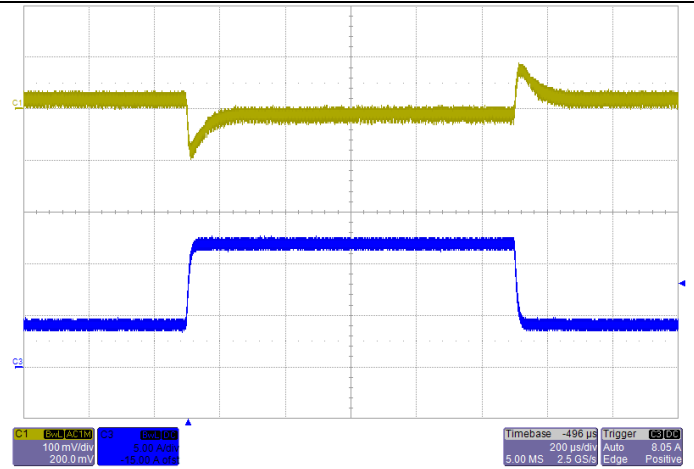
瞬态响应，输入 11V，阶跃 4A~12A~4A，输出电容 220 \mu F 蓝色：负载电流，黄色：输出纹波
