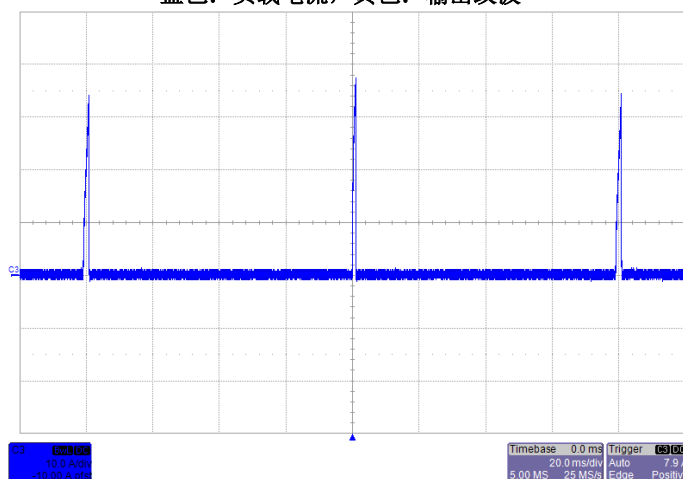
输出短路电流波形，输入电压 5V
