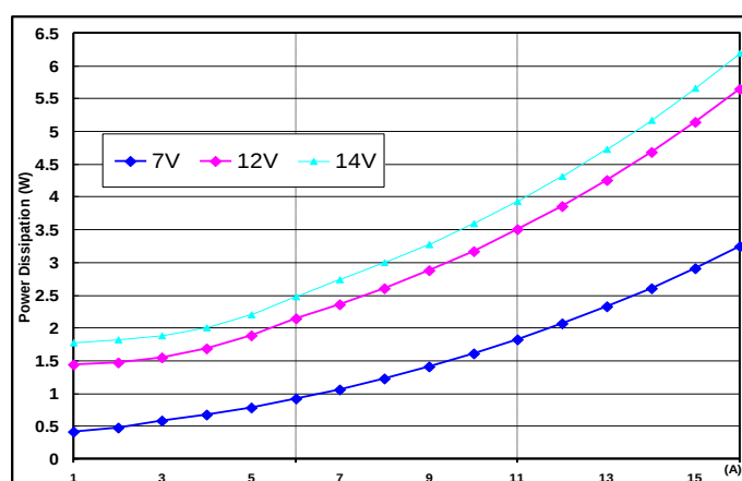
功率损耗 vs. 负载电流
