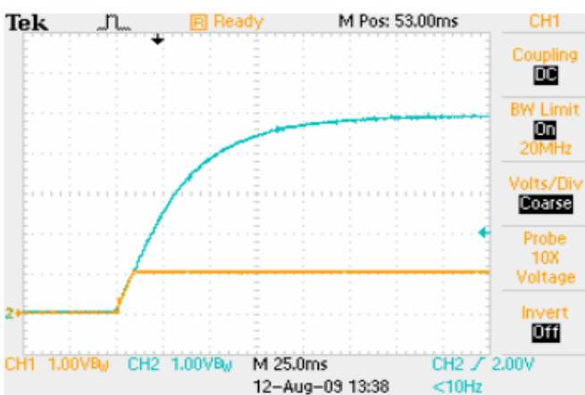
用 EasyTrack™ 控制上电过程, 控制压 5V, 负载 16A 蓝色: EasyTrack™ 控制电压 黄色: 输出电压
