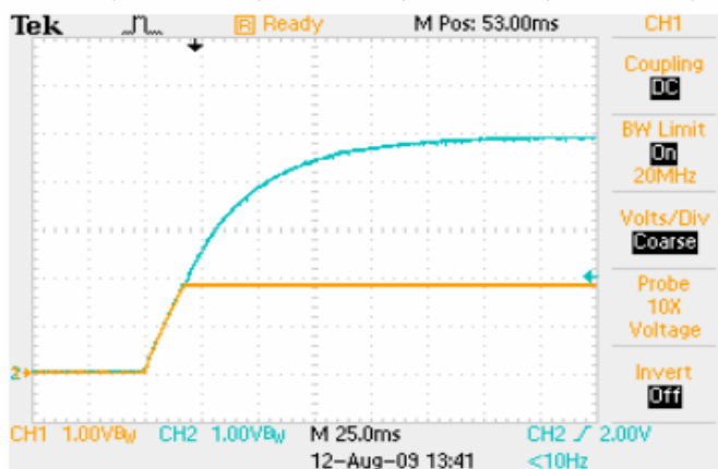
用 EasyTrack™ 控制上电过程, 控制压 5V, 负载 16A 蓝色: EasyTrack™ 控制电压 黄色: 输出电压
