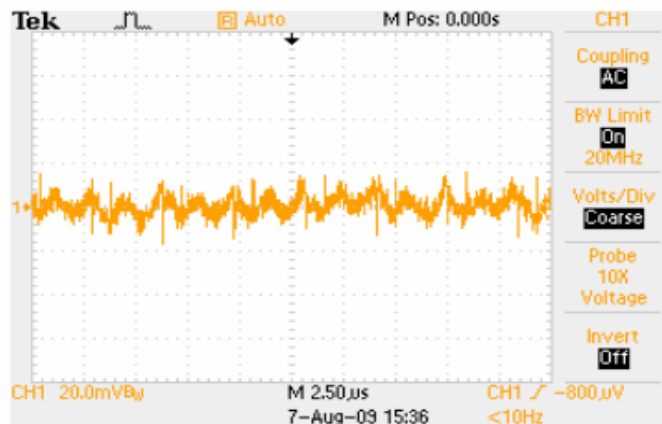
纹波与噪声: 输入 5V, 16A 负载, 5~20MHz 带宽
