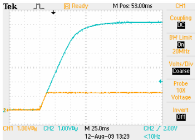
用 EasyTrack™ 控制上电过程，控制压 5V，负载 16A 蓝色：EasyTrack™ 控制电压 黄色：输出电压
