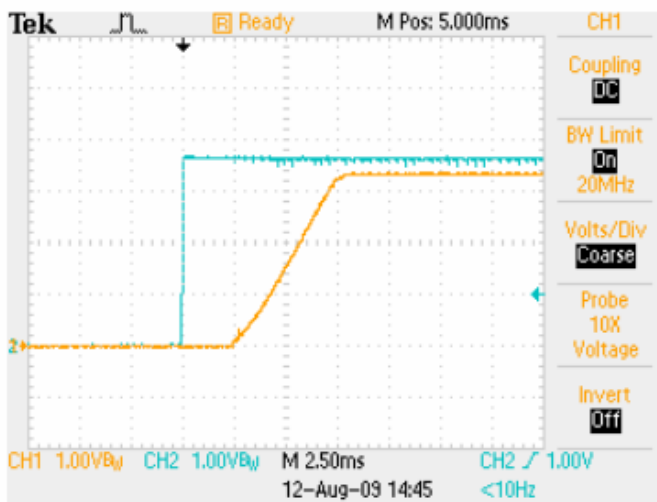
用 ON/OFF 控制上电过程，控制压 5V，负载 16A 蓝色：ON/OFF 控制电压 黄色：输出电压
