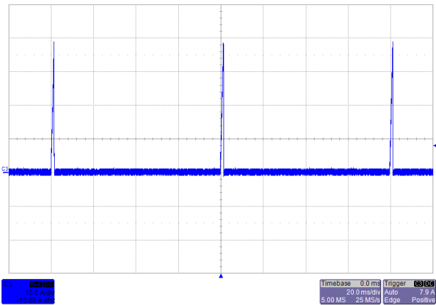
输出短路电流波形，输入电压 5V
