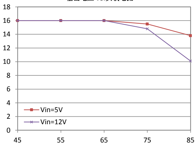
输出电流降额 (自然冷却)
