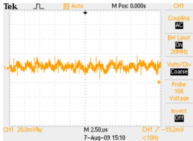
纹波与噪声: 输入 5V, 16A 负载, 5~20MHz 带宽
