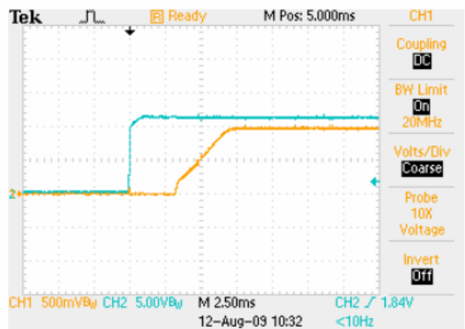
启动波形: 输入 11V, 负载 16A 黄色: 输出电压; 蓝色: 输入电压
