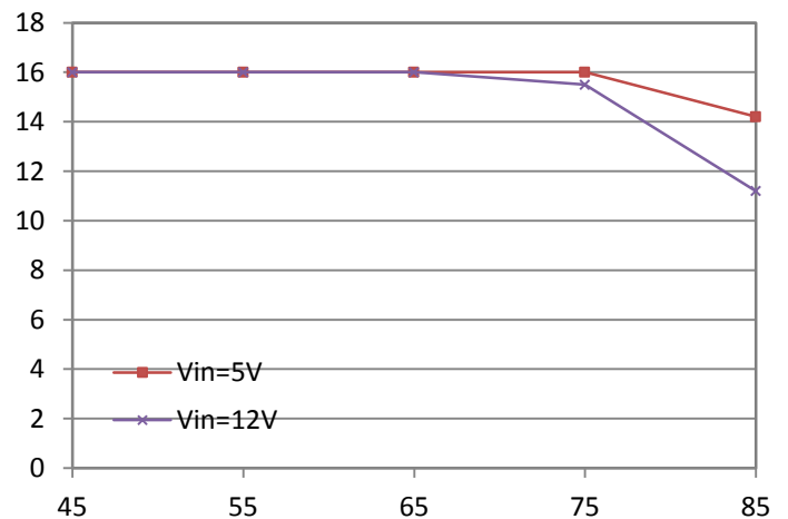
输出电流降额 (自然冷却)
