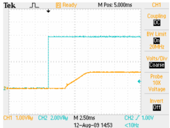
用 ON/OFF 控制上电过程，控制压 12V，负载 16A 蓝色：ON/OFF 控制电压 黄色：输出电压
