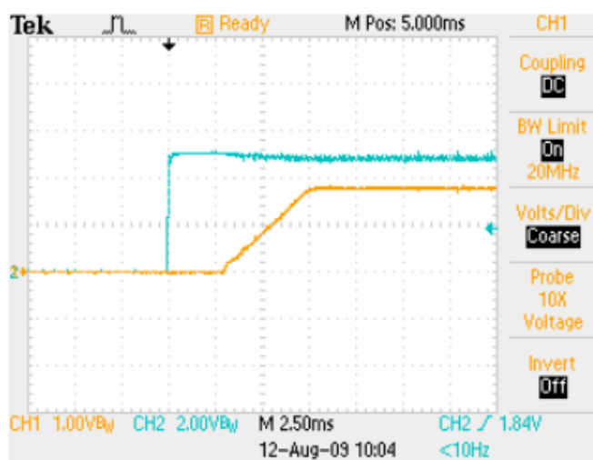
启动波形: 输入 5V, 负载 16A 黄色: 输出电压; 蓝色: 输入电压
