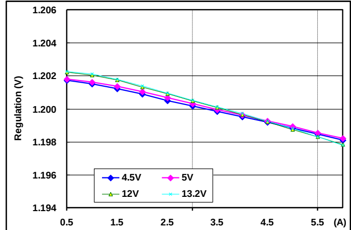
调整率 输出电压 vs. 负载电流
