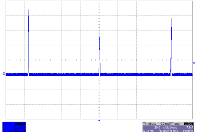
输出短路电流波形，输入电压 12V
