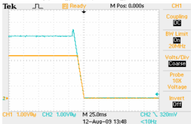
用 EasyTrack™ 控制下电过程, 控制压 5V, 负载 16A 蓝色: EasyTrack™ 控制电压 黄色: 输出电压
