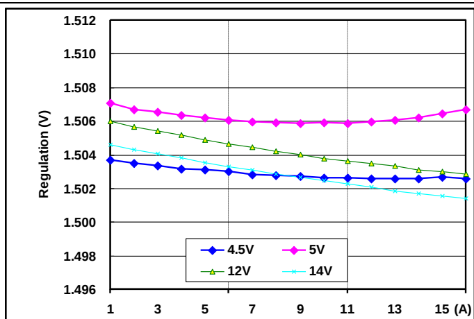
调整率 输出电压 vs.负载电流
