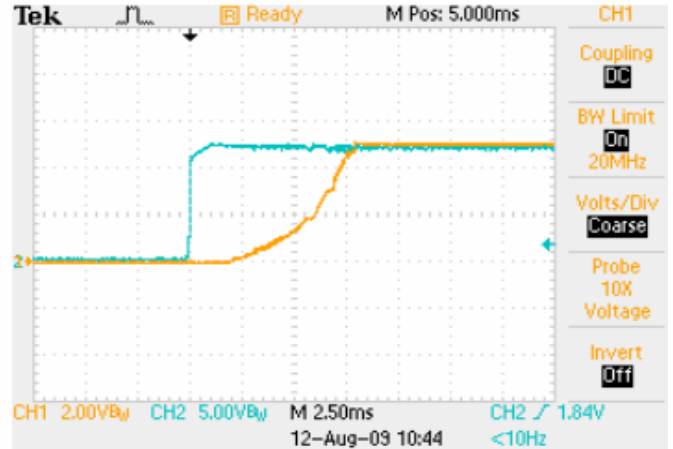
启动波形: 输入 12V, 负载 16A 黄色: 输出电压; 蓝色: 输入电压
