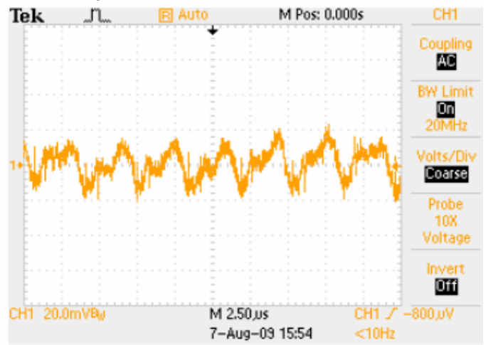
纹波与噪声: 输入 12V, 16A 负载, 5~20MHz 带宽
