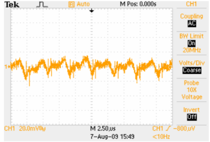
纹波与噪声: 输入 12V, 16A 负载, 5~20MHz 带宽
