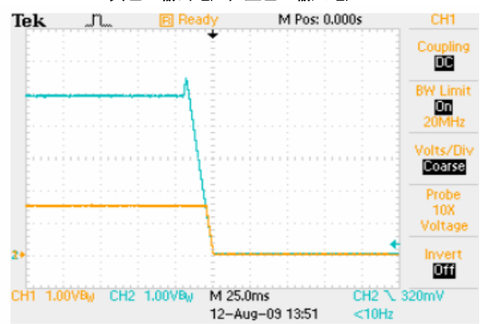
用 EasyTrack™ 控制下电过程, 控制压 5V, 负载 16A 蓝色: EasyTrack™ 控制电压 黄色: 输出电压
