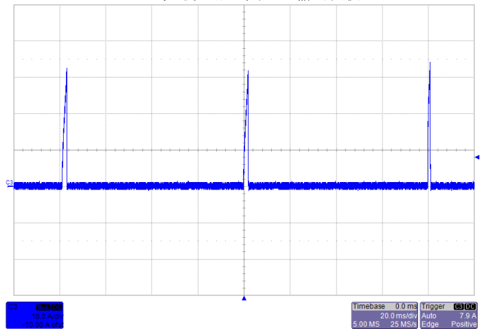
输出短路电流波形，输入电压 11V
