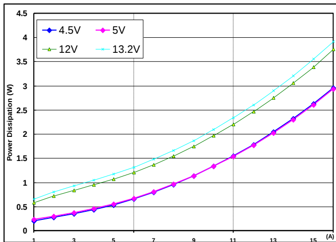
功率损耗 vs. 负载电流
