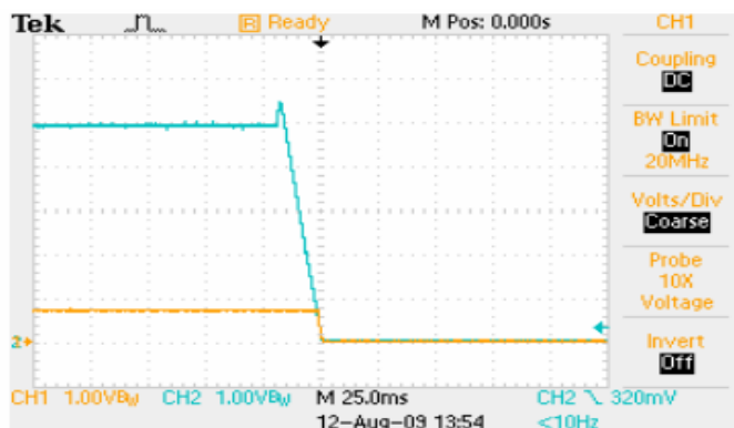
用 EasyTrack™ 控制下电过程, 控制压 5V, 负载 16A 蓝色: EasyTrack™ 控制电压 黄色: 输出电压
