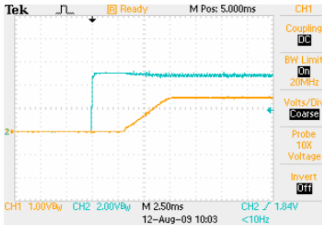
启动波形: 输入 5V, 负载 16A 黄色: 输出电压; 蓝色: 输入电压
