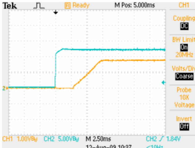
启动波形: 输入 12V, 负载 16A 黄色: 输出电压; 蓝色: 输入电压
