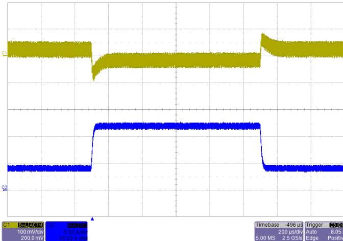
瞬态响应, 输入 12V, 阶跃 4A~12A~4A, 输出电容 220 \mu F 蓝色: 负载电流, 黄色: 输出纹波
