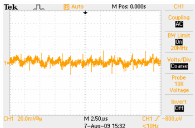
纹波与噪声: 输入 5V, 16A 负载, 5~20MHz 带宽
