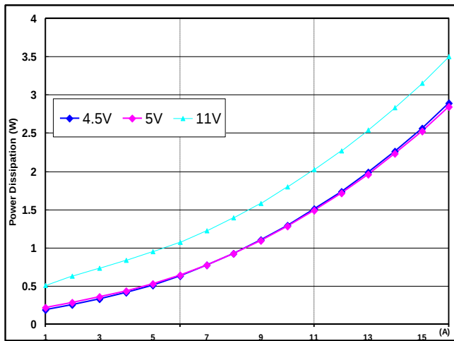
功率损耗 vs.负载电流
