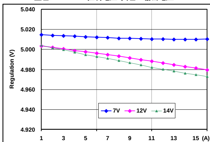
调整率 输出电压 vs. 负载电流
