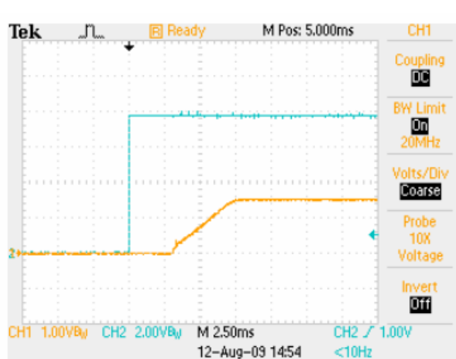
用 ON/OFF 控制上电过程，控制压 12V，负载 16A 蓝色：ON/OFF 控制电压 黄色：输出电压
