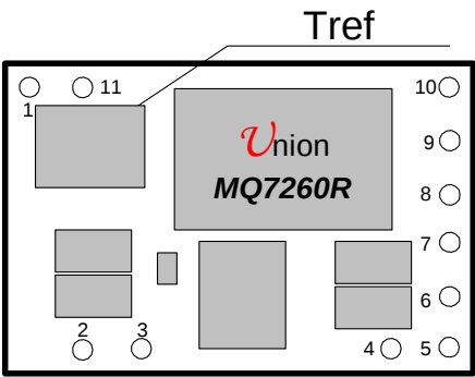
图 6，温度参考点
