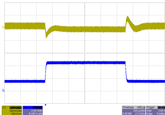
瞬态响应, 输入 12V, 阶跃 1.5A~4.5A~1.5A, 输出电容 220 \mu F 蓝色: 负载电流, 黄色: 输出纹波
