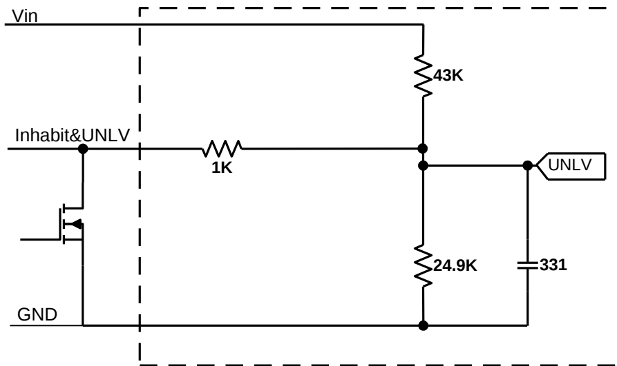
图 5, 用集电极和漏极开路晶体管实现输出的开或关
