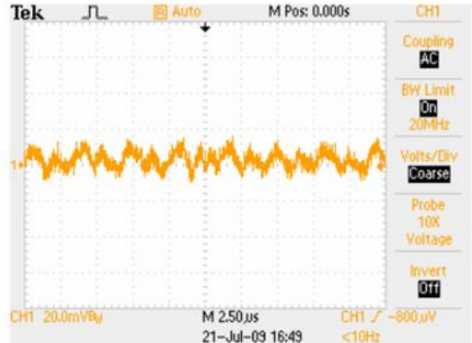
纹波与噪声: 输入 12V, 6A 负载, 5~20MHz 带宽
