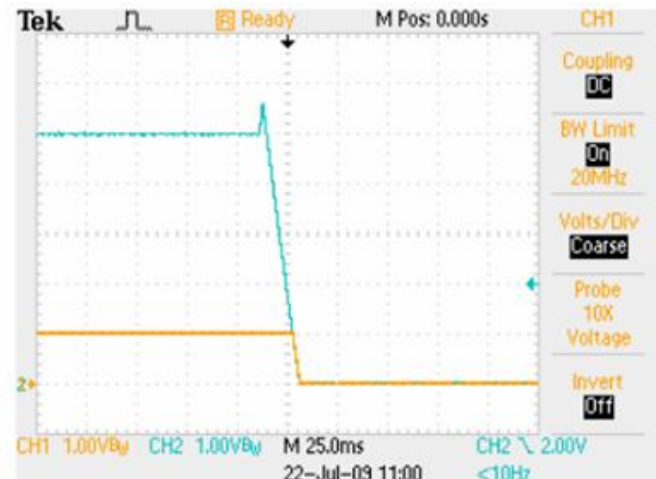
启动波形: 输入 11V, 负载 6A 黄色: 输出电压; 蓝色: 输入电压
