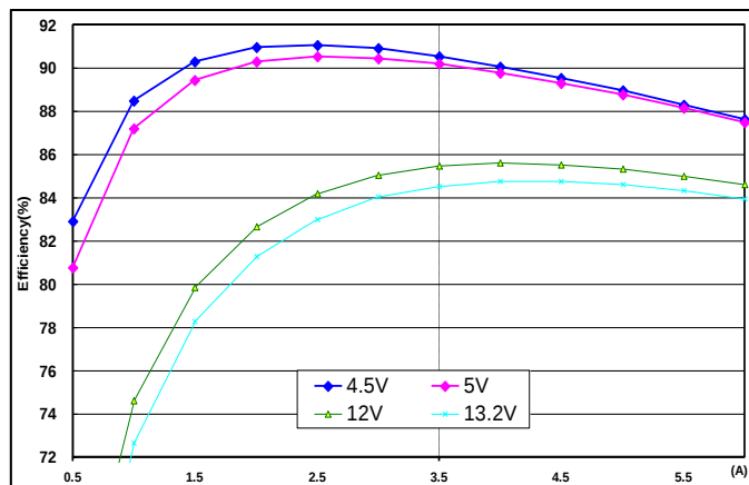
转换效率 vs.负载电流
