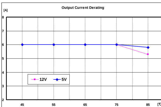
输出电流降额 (自然冷却)
