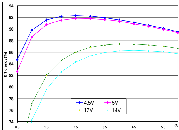
转换效率 vs. 负载电流
