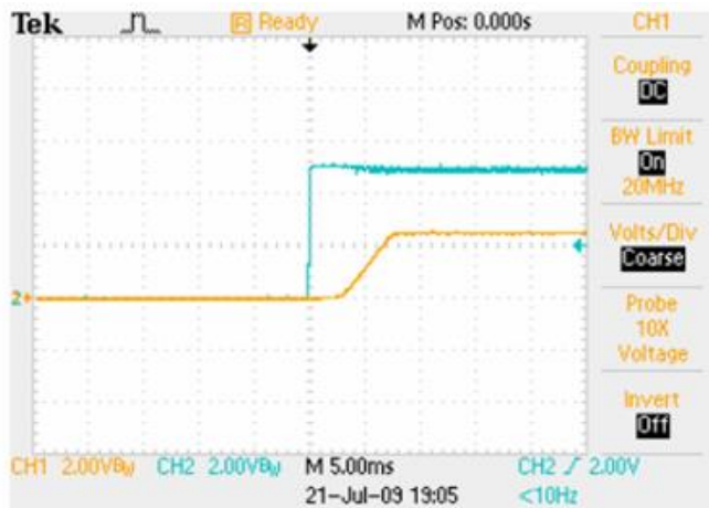
启动波形: 输入 5V, 负载 6A 黄色: 输出电压; 蓝色: 输入电压
