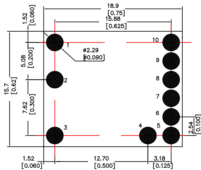
“S”焊接面
