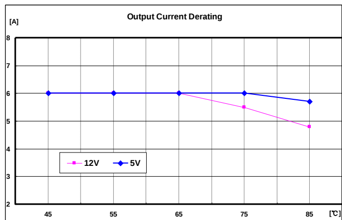
输出电流降额（自然冷却）
