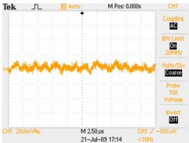
纹波与噪声: 输入 5V, 6A 负载, 5~20MHz 带宽
