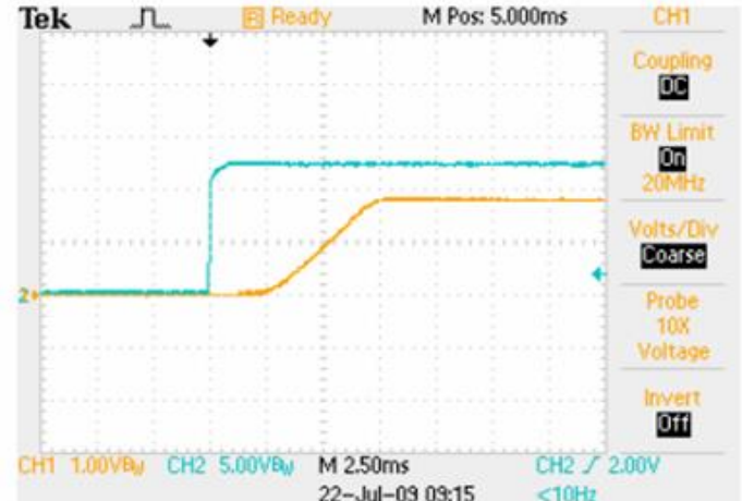
启动波形: 输入 12V, 负载 6A 黄色: 输出电压; 蓝色: 输入电压
