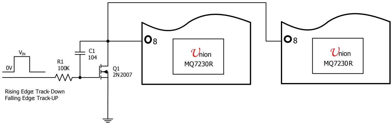
图三，使用EasyTrack™同时上电和下电电路
