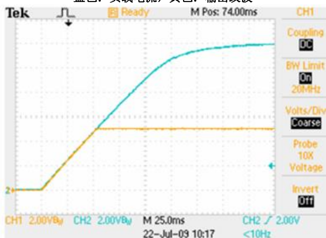
用 EasyTrack™ 控制上电过程, 控制压 12V, 负载 6A 蓝色: EasyTrack™ 控制电压 黄色: 输出电压
