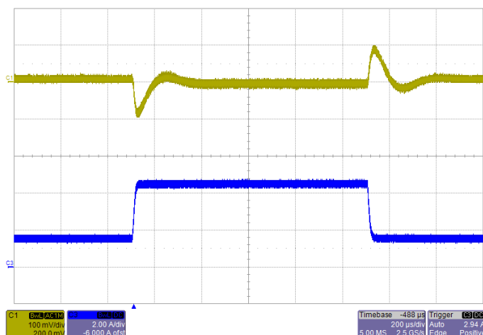
瞬态响应, 输入 5V, 阶跃 1.5A~4.5A~1.5A, 输出电容 220 \mu F 蓝色: 负载电流, 黄色: 输出纹波
