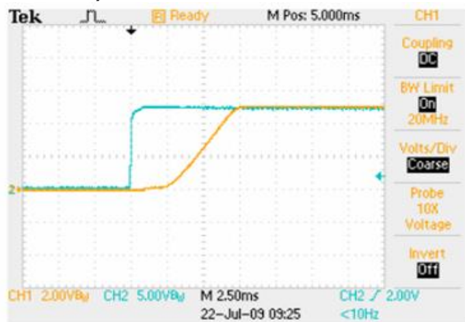
启动波形: 输入 12V, 负载 6A 黄色: 输出电压; 蓝色: 输入电压
