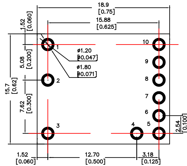
“T”焊接面
