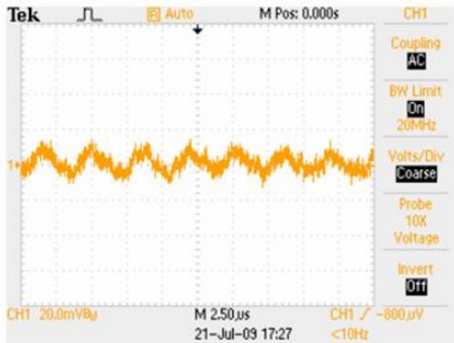
纹波与噪声: 输入 5V, 6A 负载, 5~20MHz 带宽
