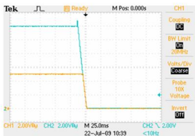
用 EasyTrack™ 控制下电过程, 控制压 12V, 负载 6A 蓝色: EasyTrack™ 控制电压 黄色: 输出电压
