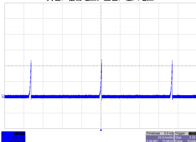
启动波形: 输入 5V, 负载 6A 黄色: 输出电压; 蓝色: 输入电压
