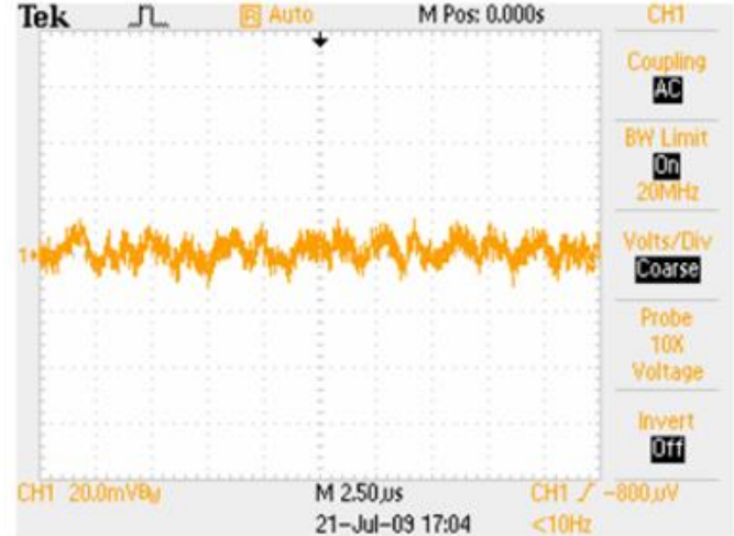
纹波与噪声: 输入 11V, 6A 负载, 5~20MHz 带宽
