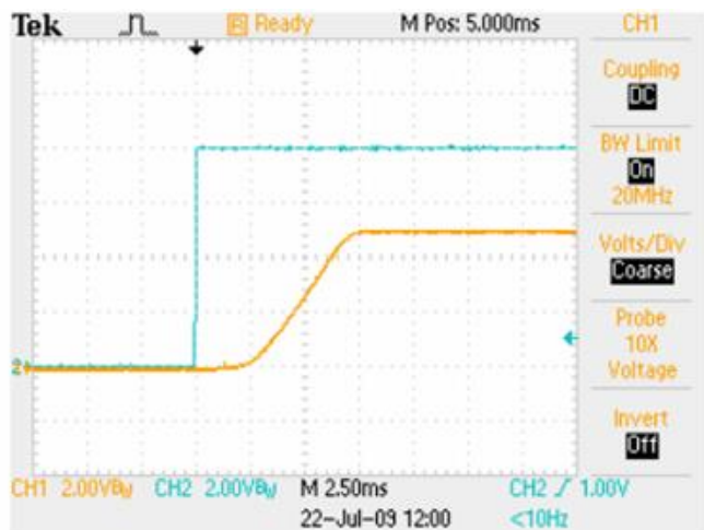
用 ON/OFF 控制上电过程, 控制压 12V, 负载 6A 蓝色: ON/OFF 控制电压 黄色: 输出电压
