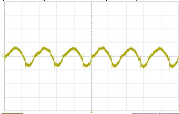
Noise V_{IN}=12V , I_O=6A , 5~20MHz Bandwidth
