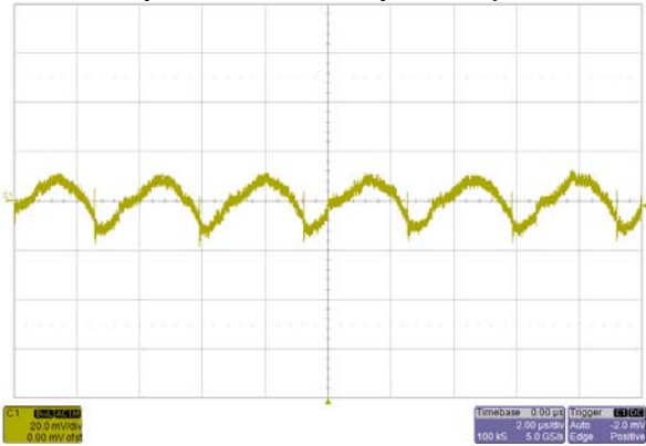
Noise V_{IN}=12V , I_O=6A , 5~20MHz Bandwidth
